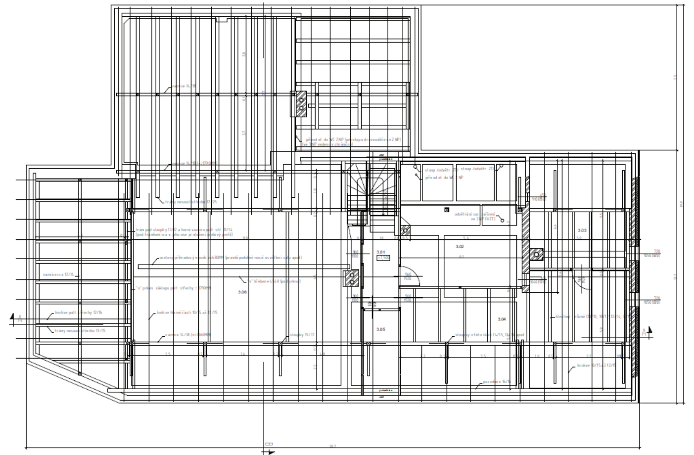
KULTURNÍ DŮM VLASTBOŘICE datum: 04/2023 objekt: STUŽKA RENOVACE PŮDORYS 3.NP. STÁVAJÍCÍ STAV
