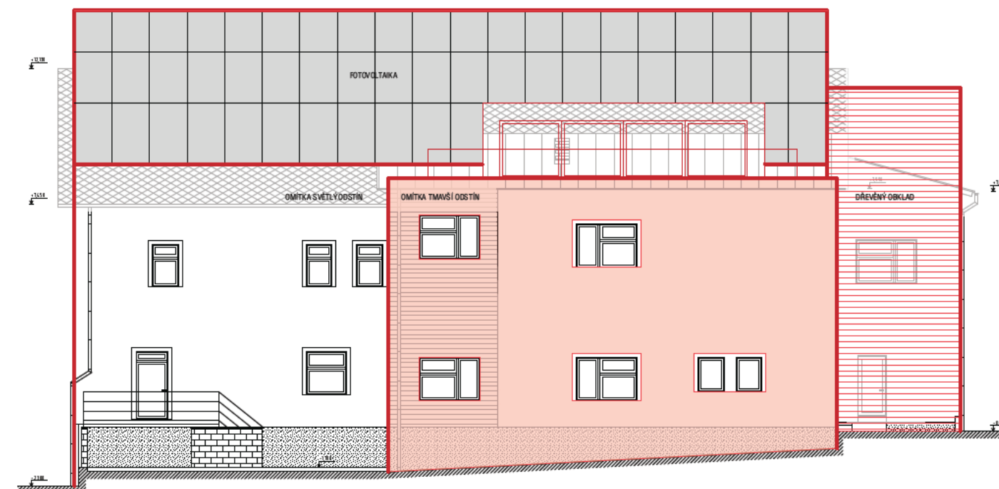
POHLED JIŽNÍ
