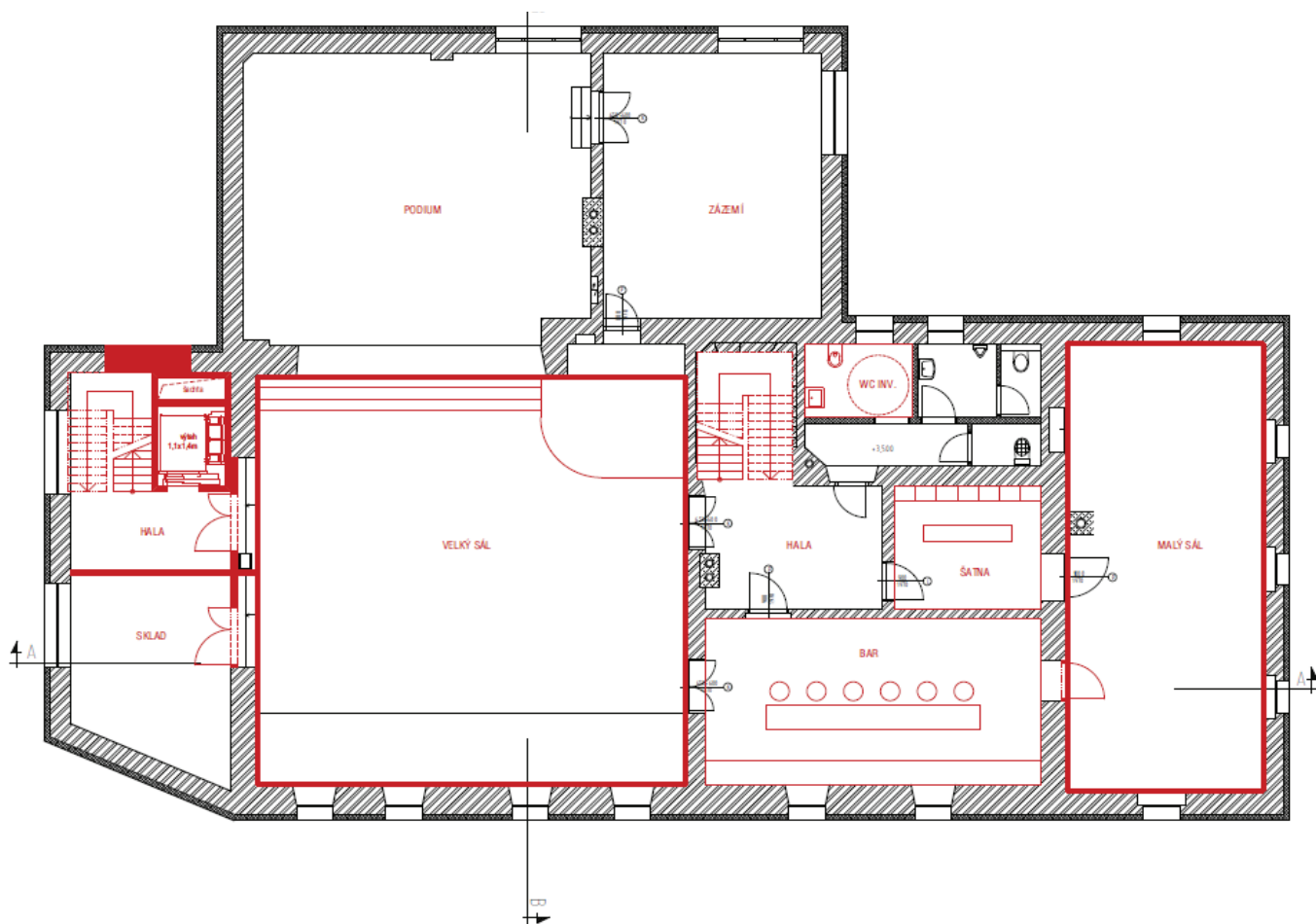
KULTURNÍ DŮM VLASTBOŘICE datum: 04/2023 objekt: STUŽKA RENOVACE PŮDORYS 2.NP. NÁVRH
