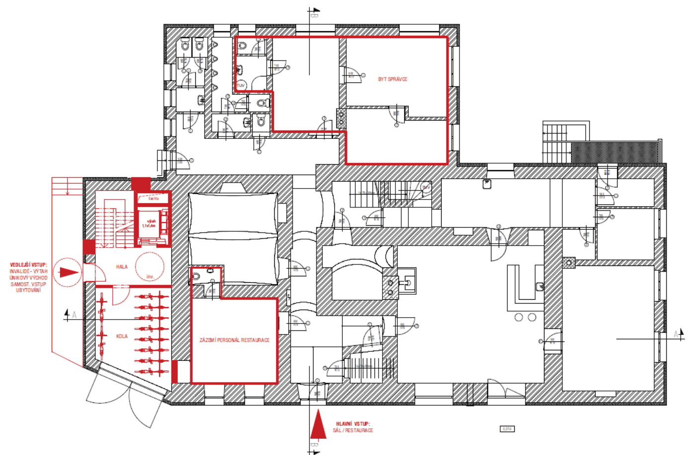
KULTURNÍ DŮM VLASTIBOŘICE OBJEKT: KULTURNÍ DŮM MÍSTO: VLASTIBOŘICE PŮDORYS 1.NP. NÁVRH
