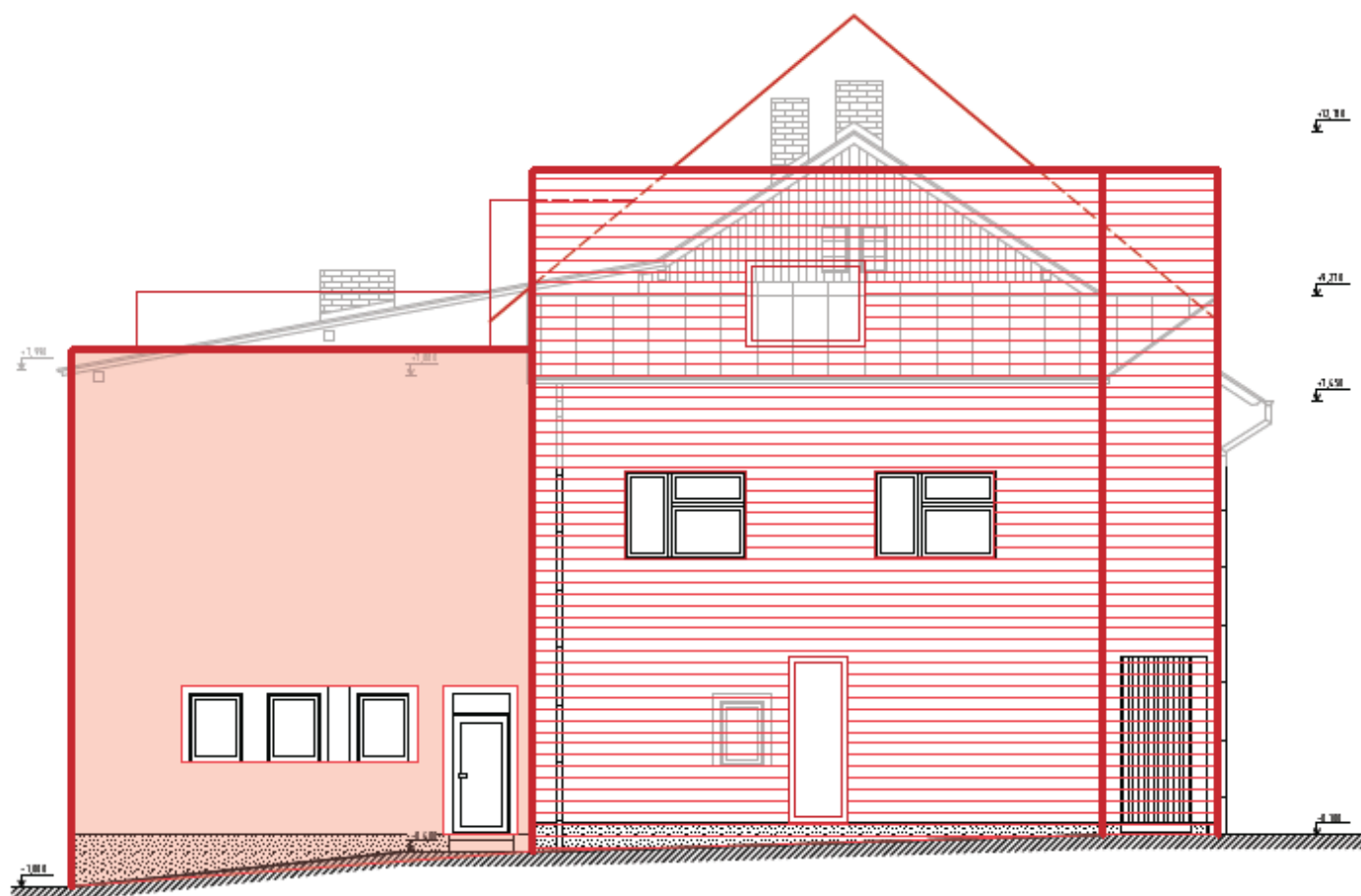
POHLED VÝCHODNÍ
