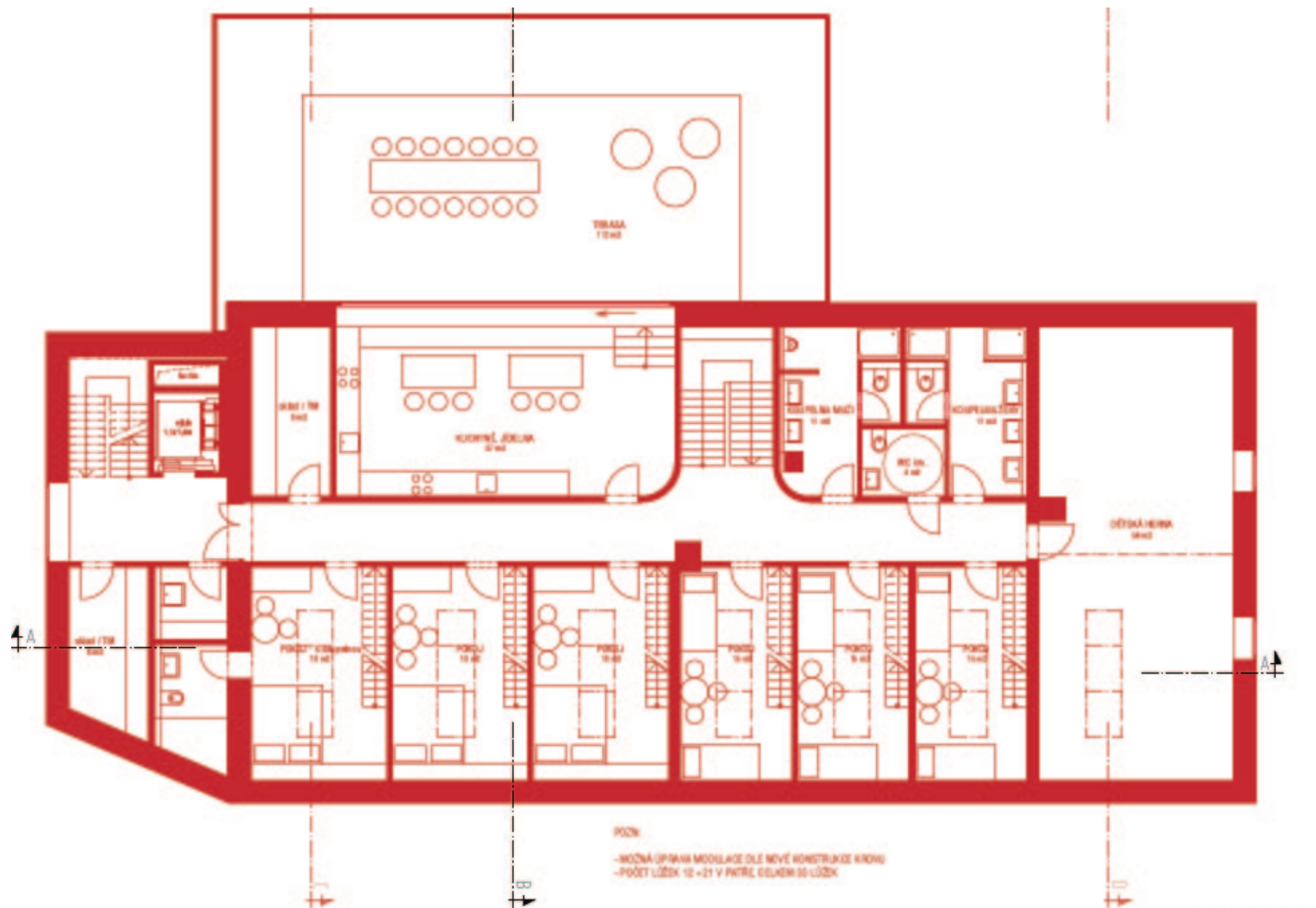
KULTURNÍ DŮM VLASTBOŘICE datum: 04/2023 objekt: STUŽKA RENOVACE PŮDORYS 3.NP. NÁVRH
