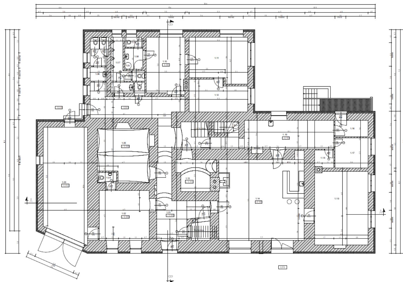
KULTURNÍ DŮM VLASTIBOŘICE OBJEKT: KULTURNÍ DŮM MÍSTO: VLASTIBOŘICE PŮDORYS 1.NP. STÁVAJÍCÍ STAV
